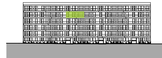
ANSICHT WEST
